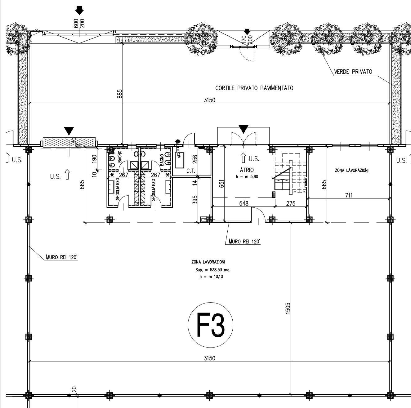
Pianta Piano Terreno
